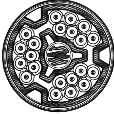
POWIERZCHNIA EMITUJĄCA ŚWIATŁO W257/AD-3 W257/AD-3 LIGHT EMITTING AREA
