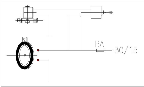
Elektrisches Diagramm
