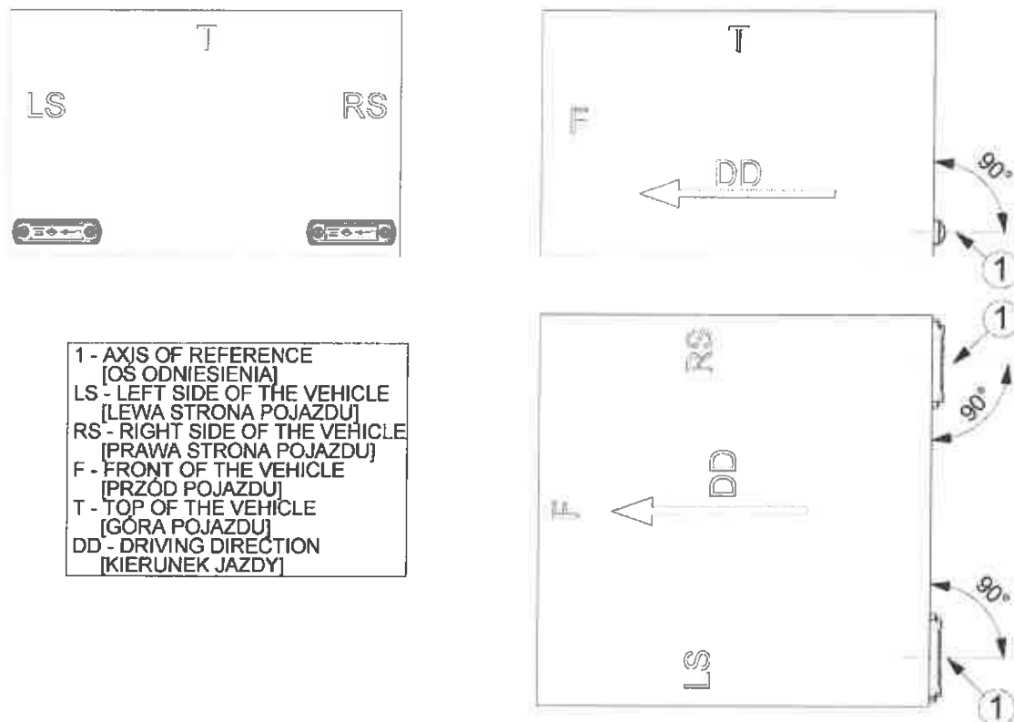
Rys. 5. Rysunek montażu lamp HOR 65G/R1 w wariantcie LD 677/GRAPHITE na pojeździe (montaż poziomy)
