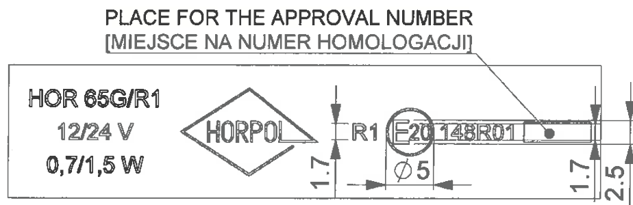
Rys. 4. Widok szczegółu ze znakiem homologacji
