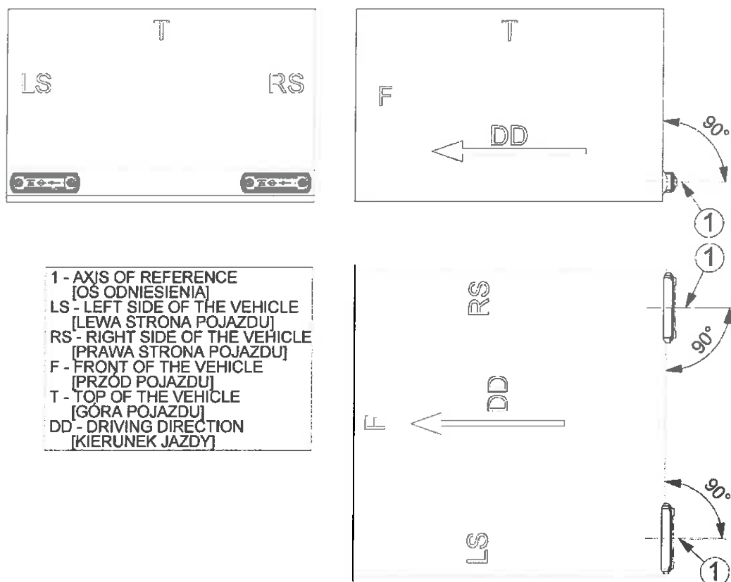
Rys. 7. Rysunek montażu lamp HOR 65G/R1 w wariantach LD 945/GRAPHITE na pojeździe (montaż poziomy)
