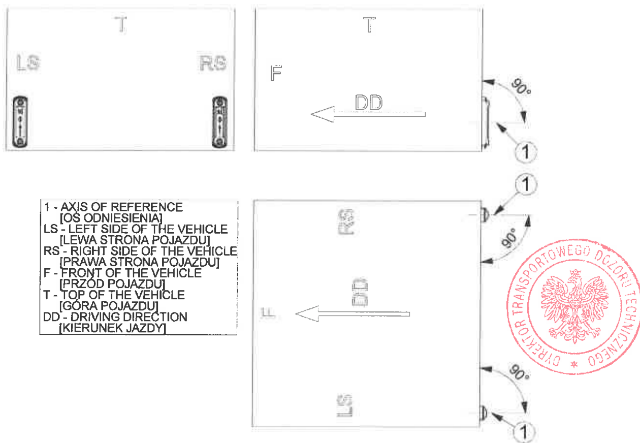
Rys. 6. Rysunek montażu lamp HOR 65G/R1 w wariantcie LD 677/GRAPHITE na pojeździe (montaż pionowy)
