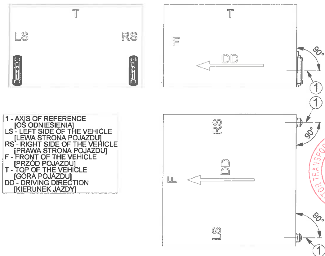
Rys. 8. Rysunek montażu lamp HOR 65G/R1 w wariantach LD 945/GRAPHITE na pojeździe (montaż pionowy)
