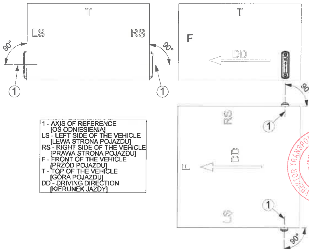
Rys. 6. Rysunek montażu lamp HOR 65G/SM1 w wariantcie LD 676/GRAPHITE na pojeździe (montaż pionowy)
