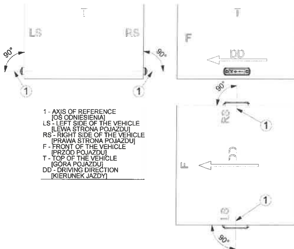
Rys. 5. Rysunek montażu lamp HOR 65G/SM1 w wariantcie LD 676/GRAPHITE na pojeździe (montaż poziomy)
