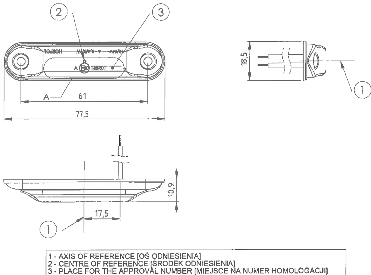
Rys. 4. Rysunek lampy HOR 88G/A zawierający miejsce na znak homologacji.
